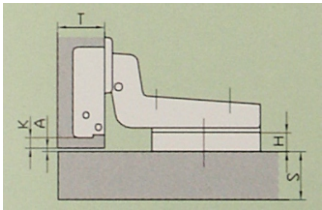
Kröpfung 15 mm, Inliegender Anschlag
