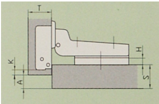
Kröpfung 8 mm, Mittelwandanschlag
