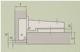
Kröpfung 0 mm, Eckanschlag
