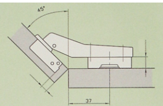
Stollenanschlag 45°
