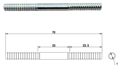
Verbindungsbolzen Ø 5 x 70 mm Eisen verzinkt
