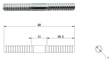
Verbindungsbolzen Ø 5 x 50 mm Eisen verzinkt
