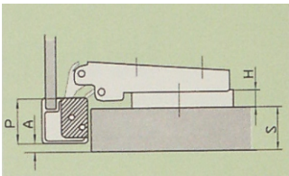
Kröpfung 0 mm, Eckanschlag
