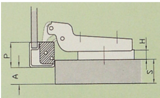
Kröpfung 8 mm, Mittelwandanschlag
