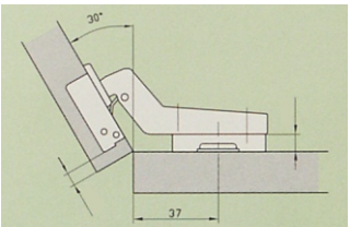
Stollenanschlag 30°
