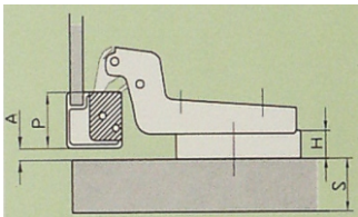
Kröpfung 15 mm, Inliegender Anschlag
